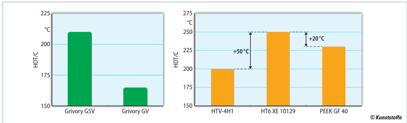
Bild 2. Der neue Polyamidtyp G5V hat mit 210°C eine deutlich erhöhte Wärmeformbeständigkeit als die herkömmliche GV-Variante. Das PPA Grivory HT6 hat nicht nur eine um 50°C höhere Wärmeformbeständigkeit als herkömmliche PPA's, sondern schlägt auch den Hochleistungskunststoff PEEK
