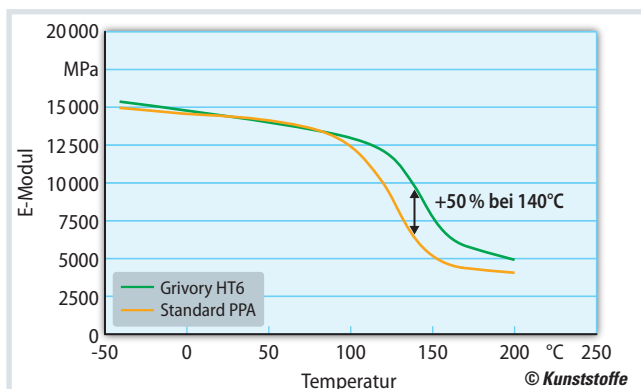
Bild 4. Bei 140°C hat Grivory HT6 gegenüber Standard PPA eine rund 50% höhere Steifigkeit
