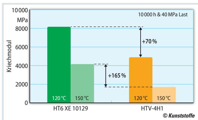
Bild 3. Grivory HT6 hat eine deutlich höhere Kriechbeständigkeit als herkömmliche PPA's
