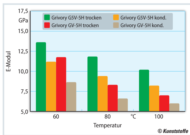
Bild 1. Grivory G5V weist im Vergleich zum bereits bekannten Grivory GV zwischen 60°C und 100°C deutliche bessere mechanische Eigenschaften auf (Quelle: Ems-Chemie)
